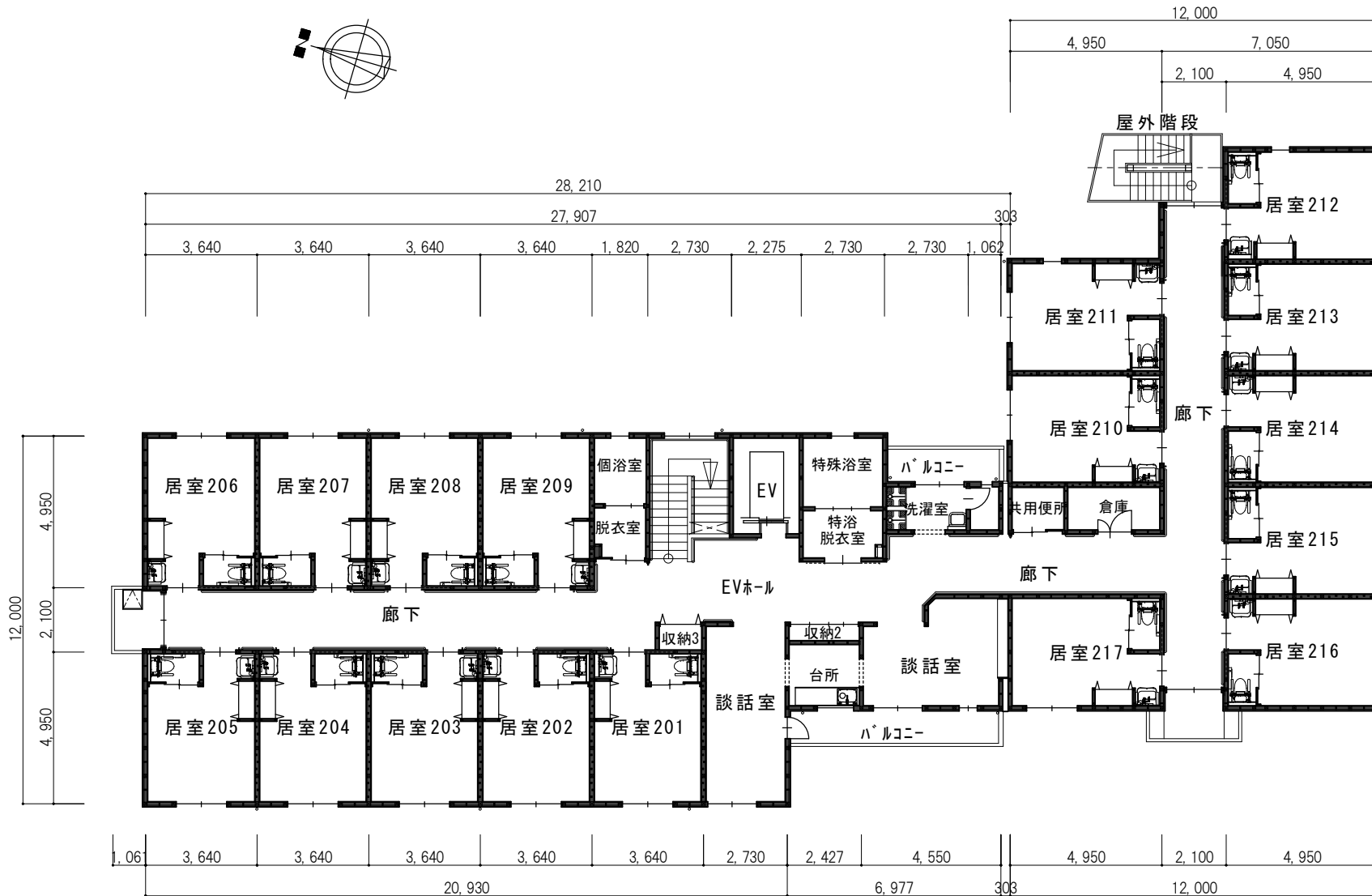
2階平面図 S=1/200
